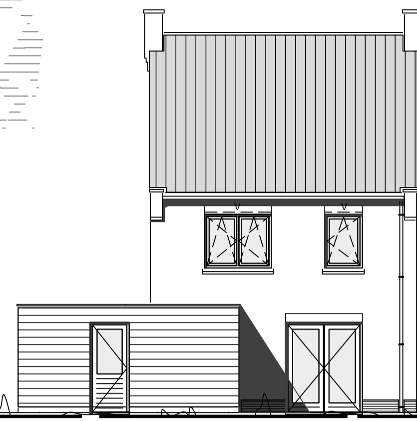
achtergevel
