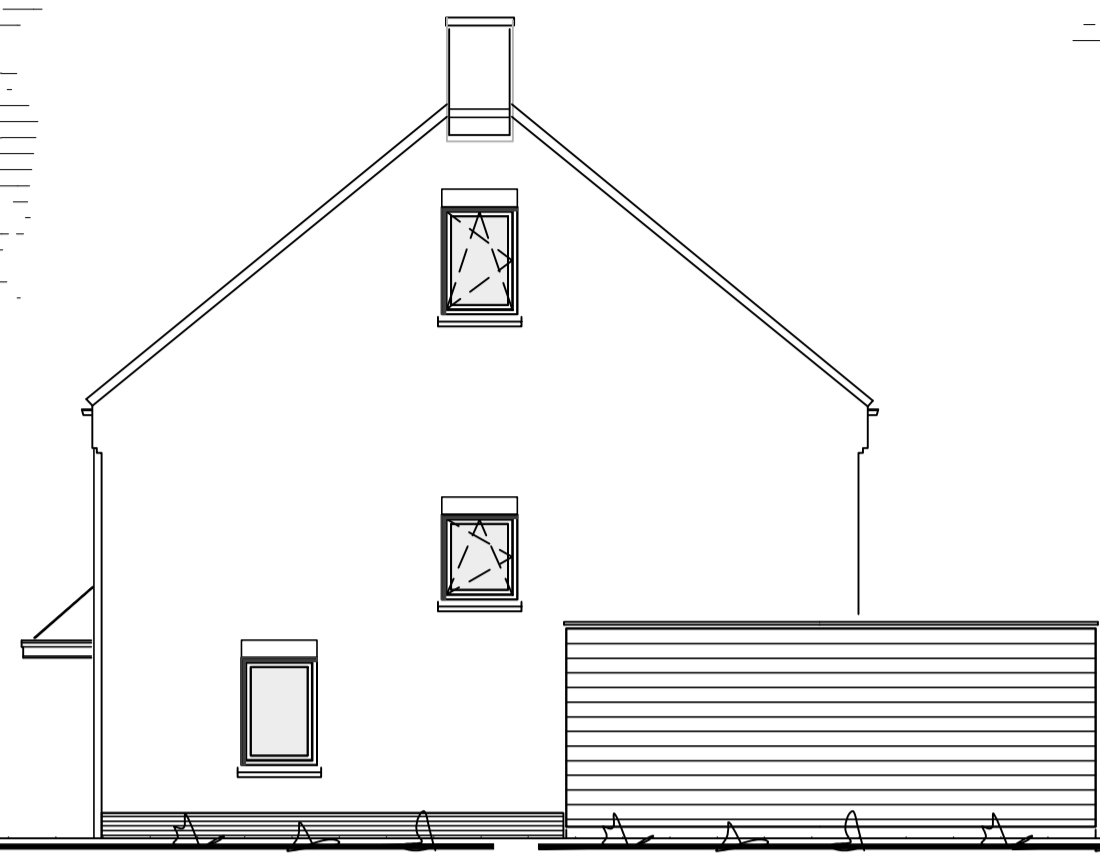
rechter zijgevel
