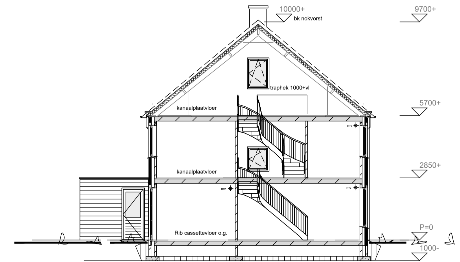
doorsnede
