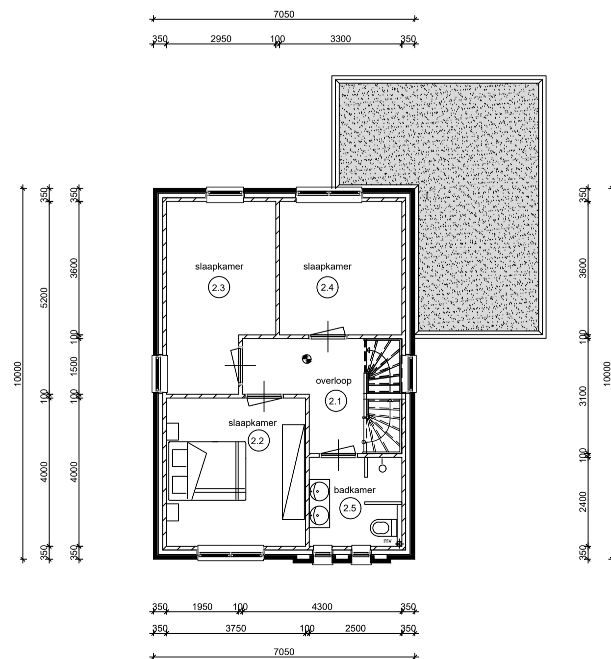
verdieping
